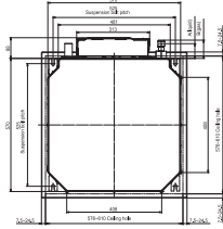
SLZ - 4-cestné kazetové jednotky, chlazení / topení, SLZ-M15 - 60FA
