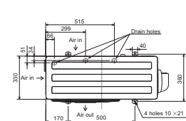
MUZ - invertorové venkovní jednotky, chlazení / topení, MUZ-EF50VG
