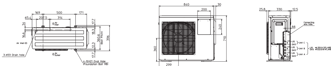
MXZ-3F54/68VF3
